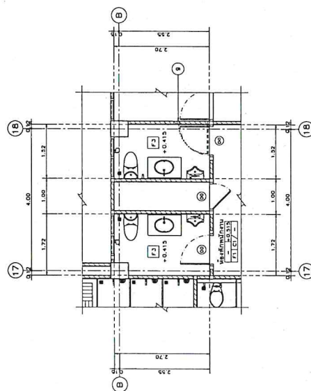
แปลนพื้นห้องน้ำคนพิการ 1
